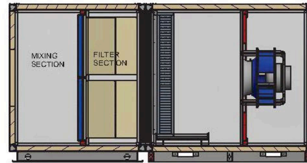
A-A (1 : 26)
